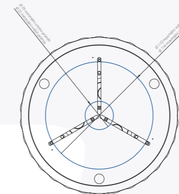
Rozměry se středícími kolíky ve vnější poloze
