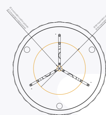
Rozměry se středícími kolíky ve vnitřní poloze
