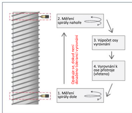
Vyrovnání na závitu Měření spirály na závitě hřídele
