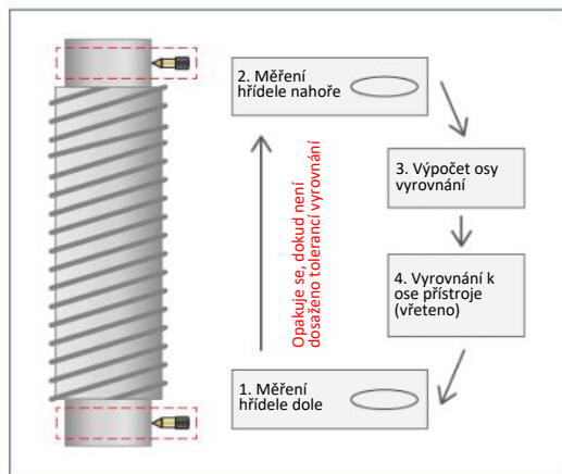
Vyrovnání na hřídeli Měření kruhovitosti na hřídeli
